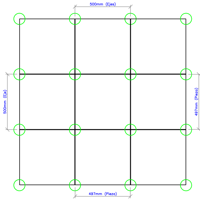
DETALLE EN PLANTA
